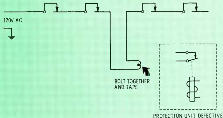
INTERLOCK CIRCUITS
